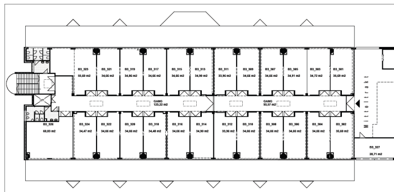
GRUNDRISS 2.OG ORDERBEREICH 1:200
